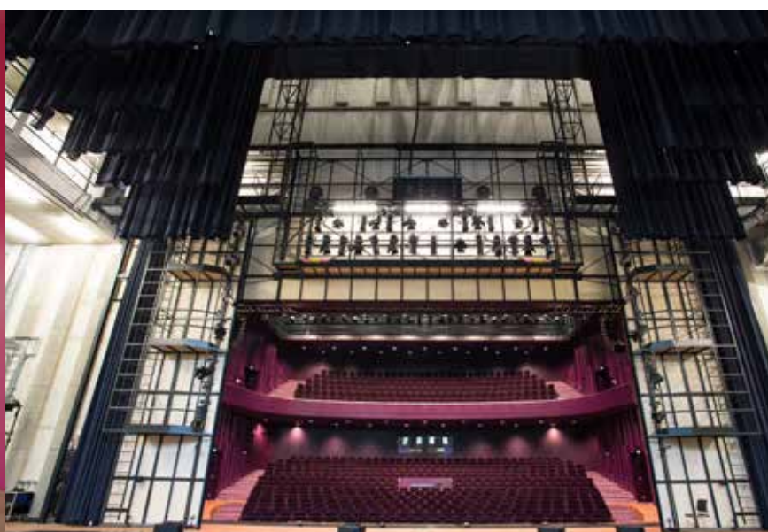
Toneelopening met manteaus en portaalbrug. | FOTO: © MARTIJN SCHOLTENS |
